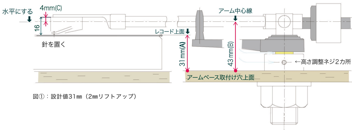
トーンアーム取付・寸法確認図
